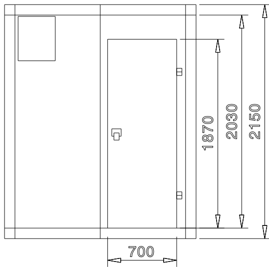
Zij aanzicht
